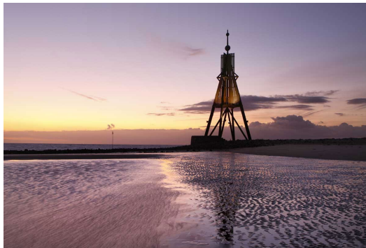
Bildtafel – Bsp. Kugelbake - Cuxhaven
